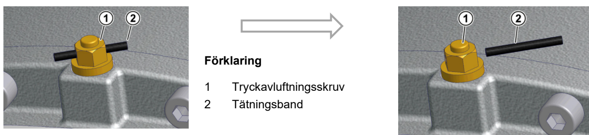
Bild 21: Aktivera tryckavluftningsskraven
