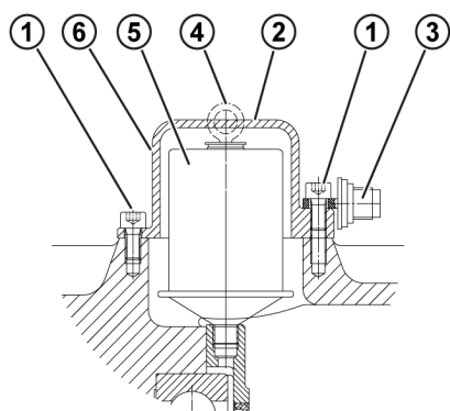
Bild 28: Byta automatisk smörjpatron vid monterad standardmotor
