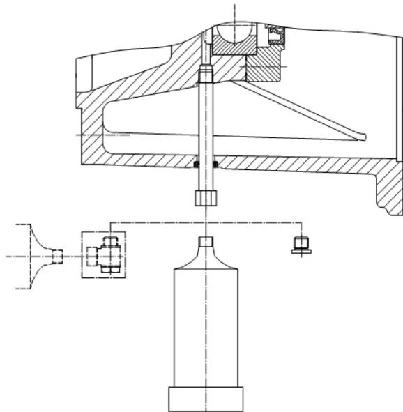
Bild 23: Montera fettuppsamlingsbehållare
