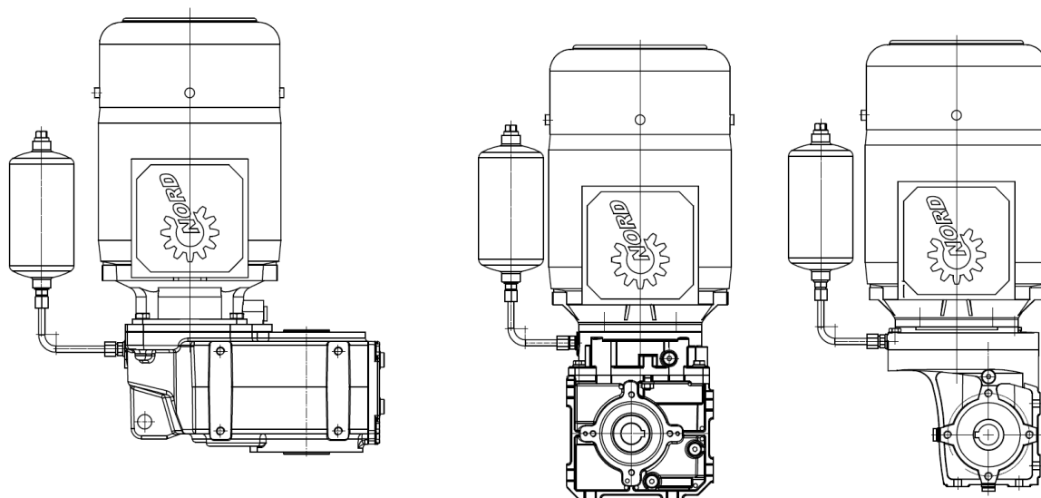
Bild 19: Oljeexpansionskärlets position
