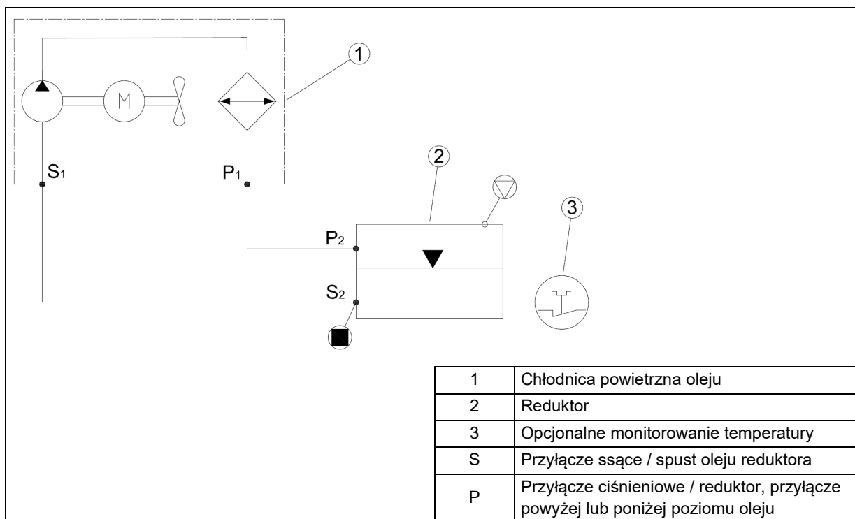
Rysunek 17: Podłączenie chłodnicy powietrznej oleju
