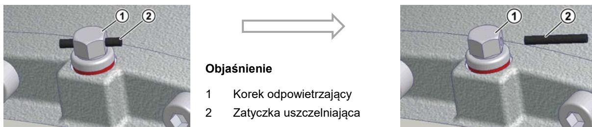
Rysunek 20: Aktywacja korka odpowietrzającego
