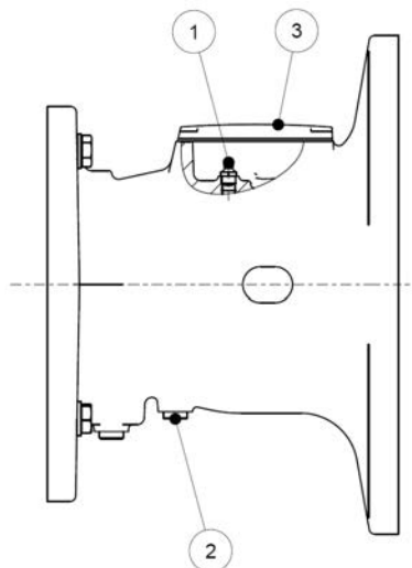
Rysunek 27: Smarowanie adaptera IEC/NEMA AI i AN z opcją BRG1
